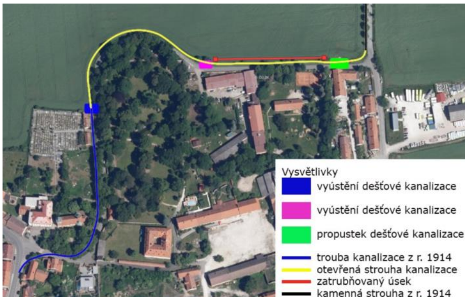
Schéma zatrubnění v ulici Pode Zděmi.
